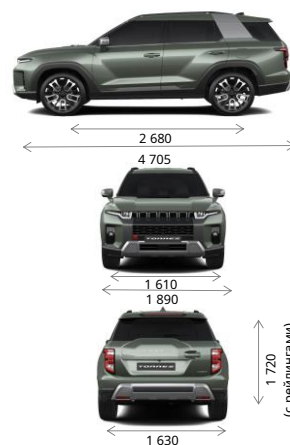
Размеры, мм
